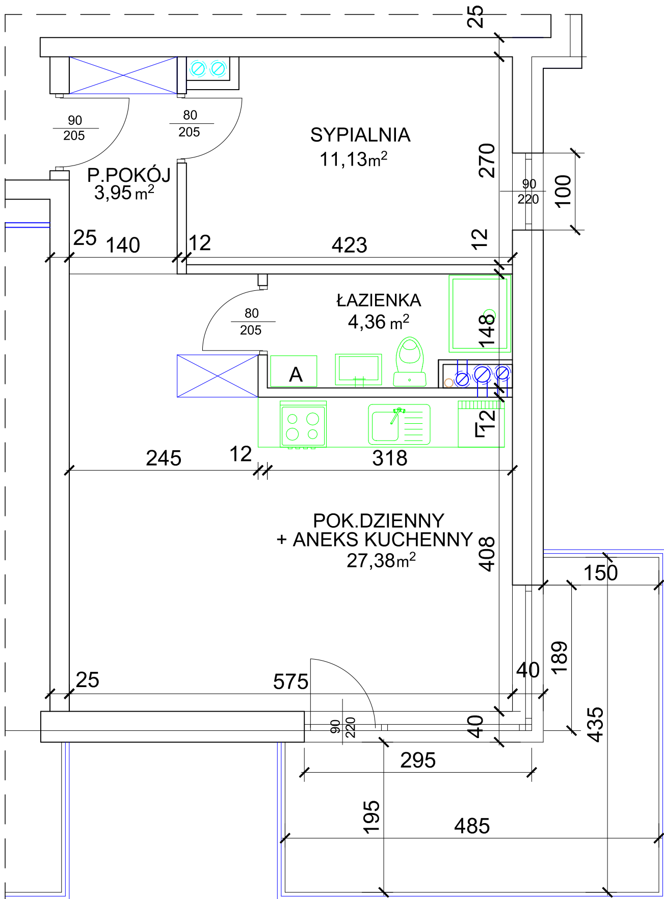
SKALA 1:50 MIESZKANIE D16.2 L II PIĘTRO 46,82 m 2
