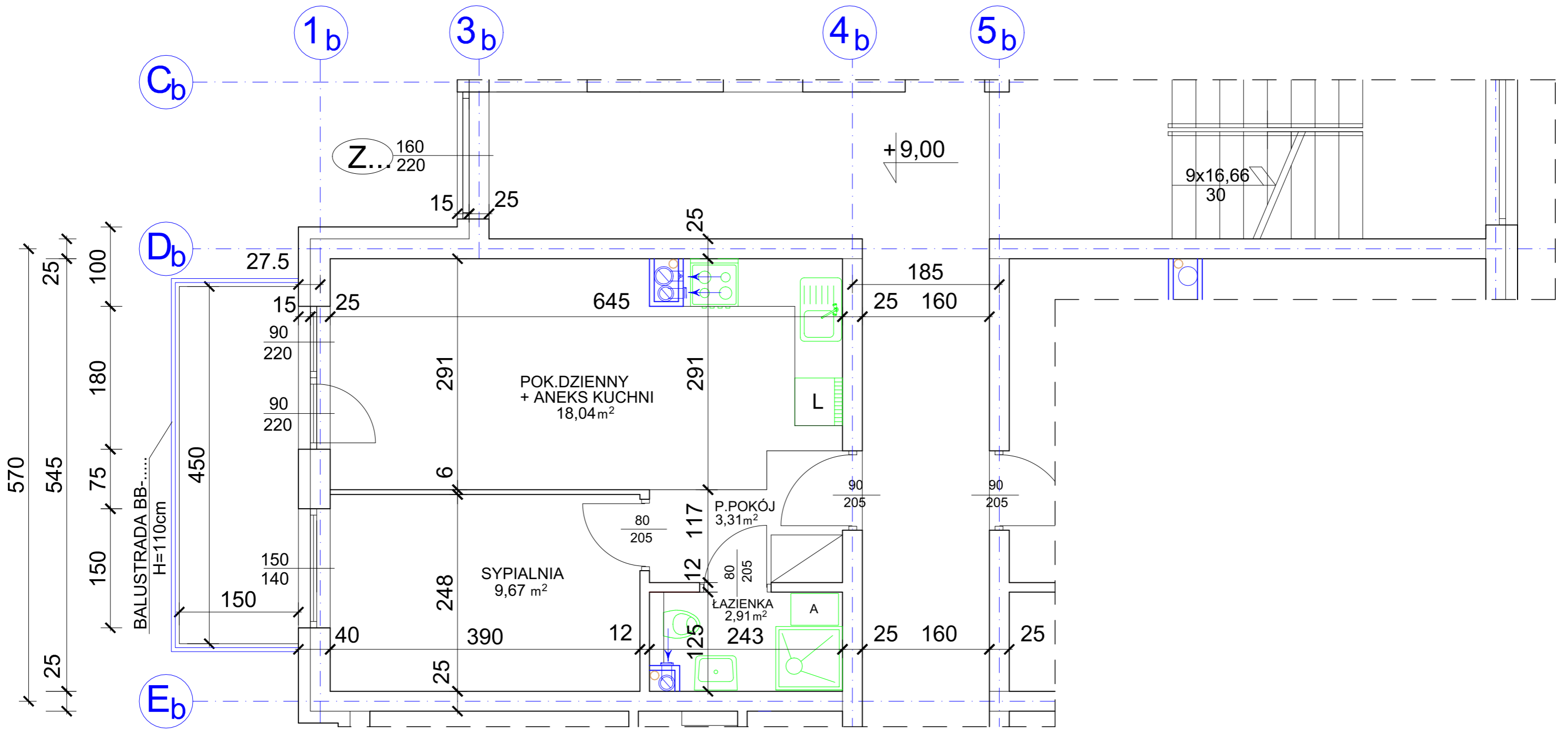
MIESZKANIE B3.3 33,93 m 2 L SKALA 1:50 III PIĘTRO
