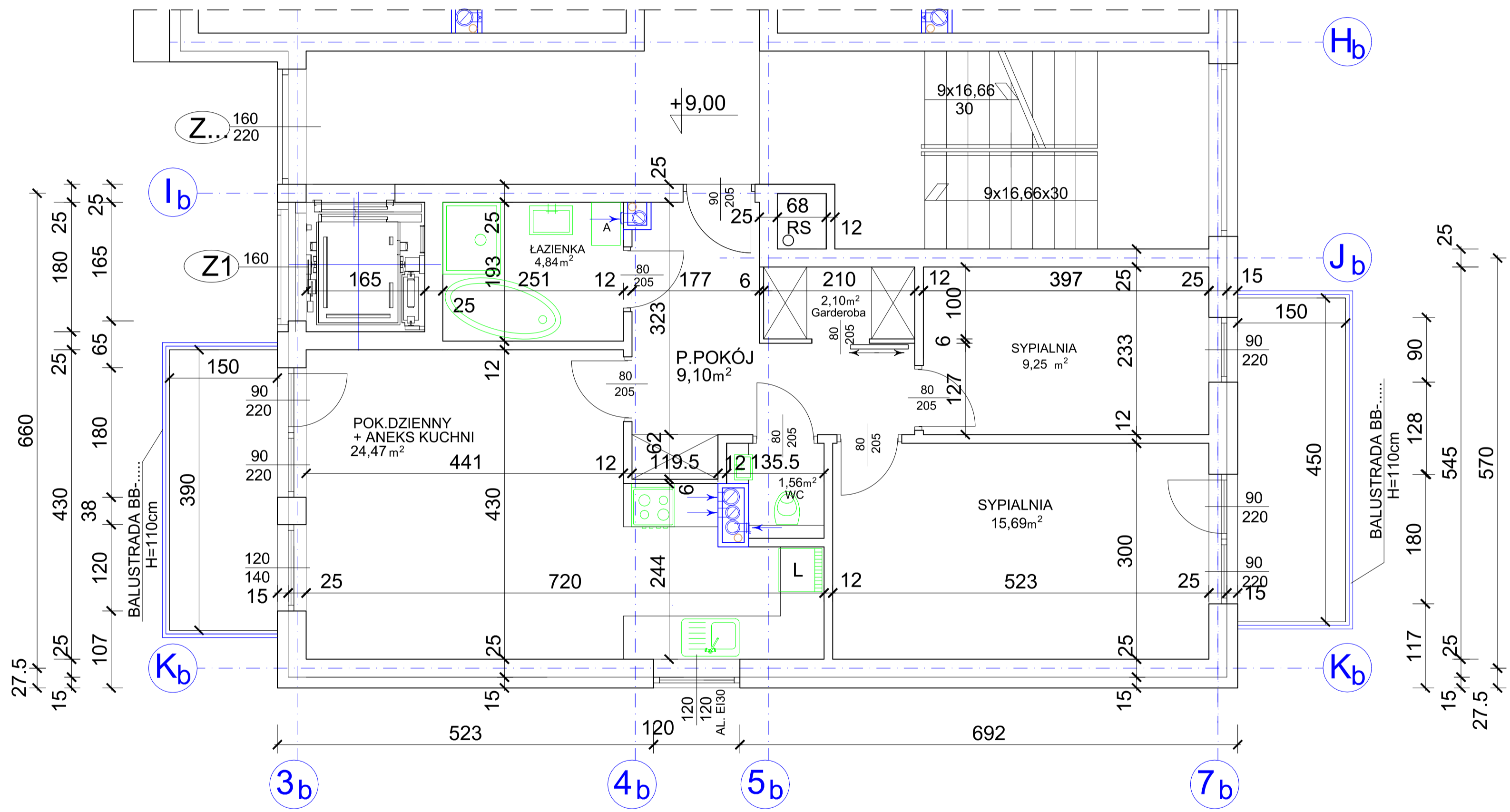
MIESZKANIE B11.3 67,01 m 2 P SKALA 1:50 III PIĘTRO
