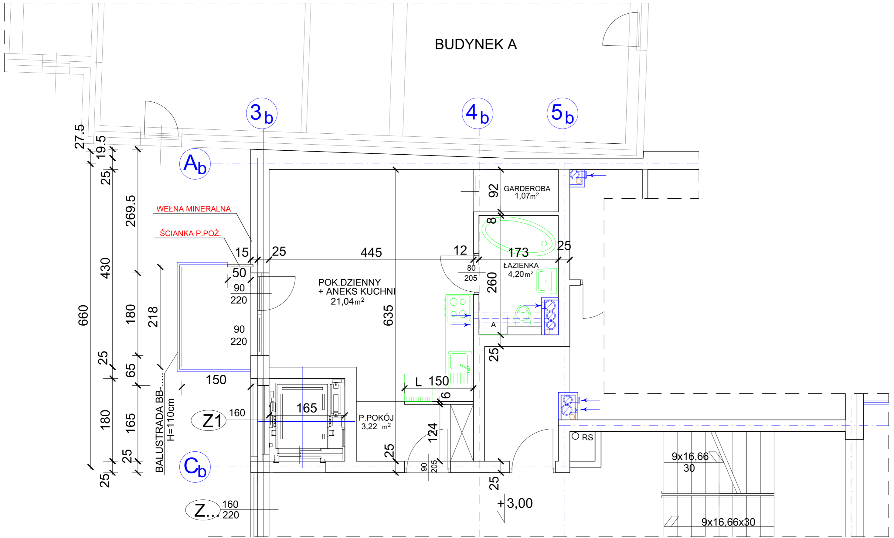
MIESZKANIE B1.1 29,53 m 2 L
