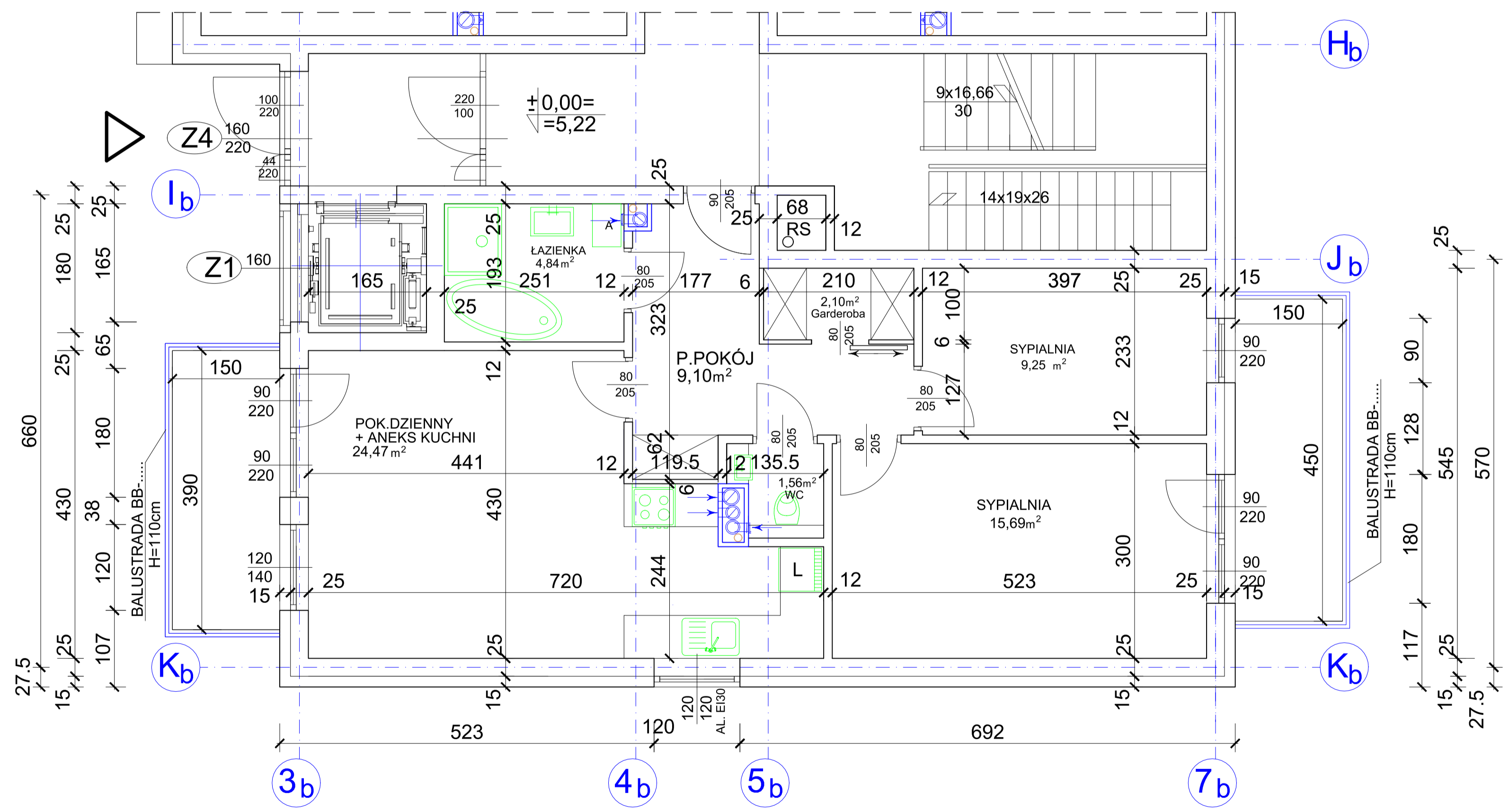
MIESZKANIE B11.0 67,01 m 2 P SKALA 1:50 PARTER
